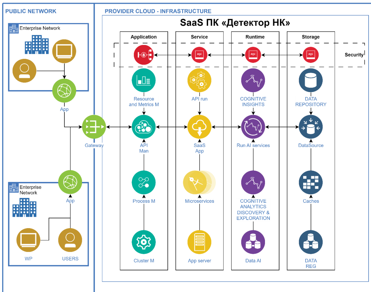
Рисунок 3.1.1 Схема серверной архитектуры SaaS ПК «Детектор НК запрещенных объектов»
